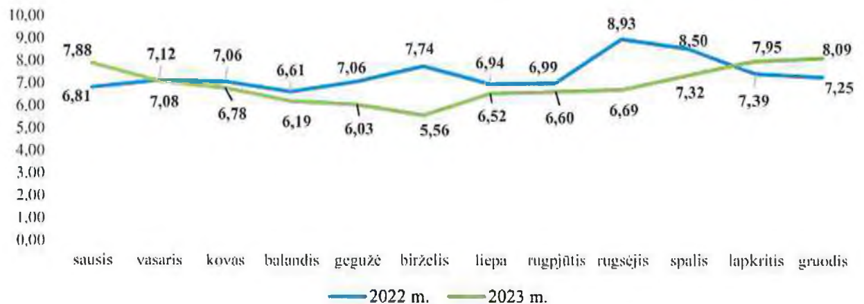
10 paveikslas. 2022 m. ir 2023 m. karšto vandens kainų gyventojams palyginimas (be PVM), Eur/m 3
