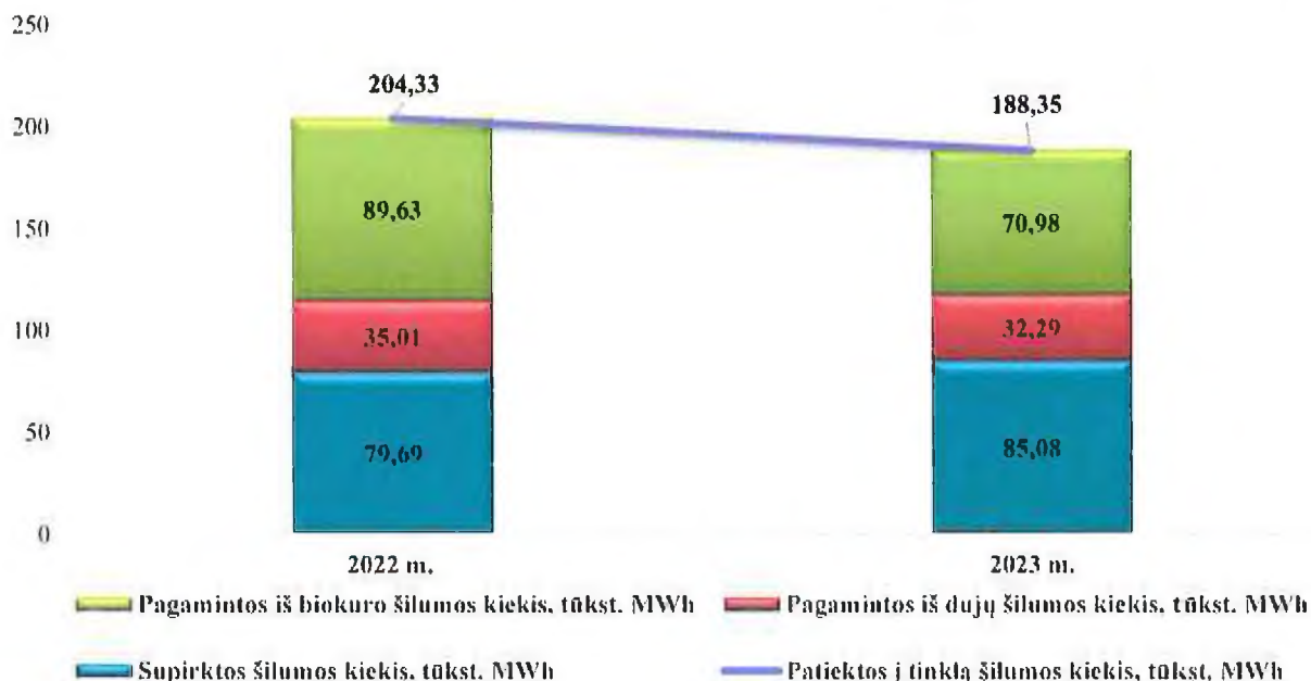
11 paveikslas. 2022 m. ir 2023 m. pagamintos ir supirktos iš NŠG šilumos kiekiai, tūkst. MWh
