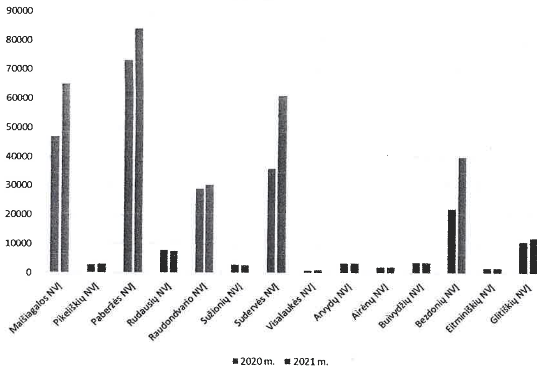
6 pav. 2020 m. ir 2021 m. išvalytų nuotekų kiekiai (m 3 )
