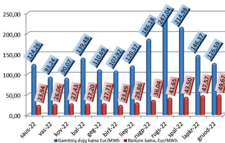
5 pav. UAB „Kaišiadorių šiluma“ vidutinės gamtinių dujų kainos (su transportavimo, skirstymo, SGD terminalo saugumo dedamąją ir galios mokesčiu) ir biokuro kainos dinamika 2022 m.
