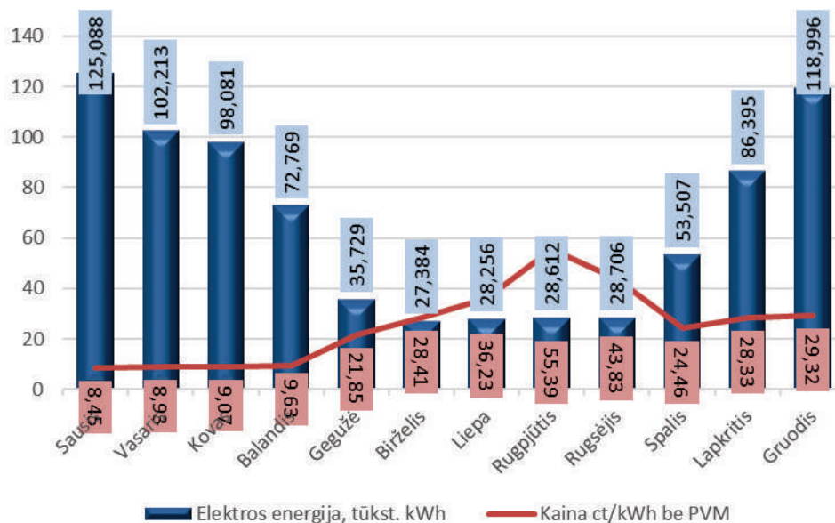
8 pav. UAB „Kaišiadorių šiluma“ 2022 m. šilumos tiekimo veiklai įsigytos elektros energijos kiekiai ir kainos ct/kWh dinamika.
