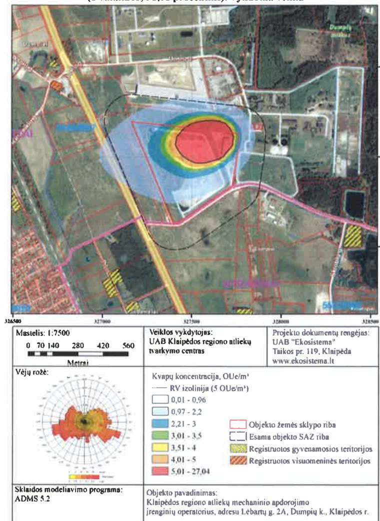
2 pav. Mechaninio apdorojimo įrenginių skleidžiamų kvapų sklaida aplinkos ore
