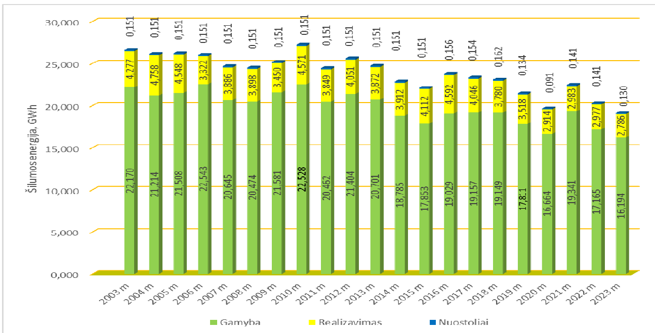
10 pav. UAB „Šakių šilumos tinklai“ 2003 – 2023 m šilumos gamyba.
