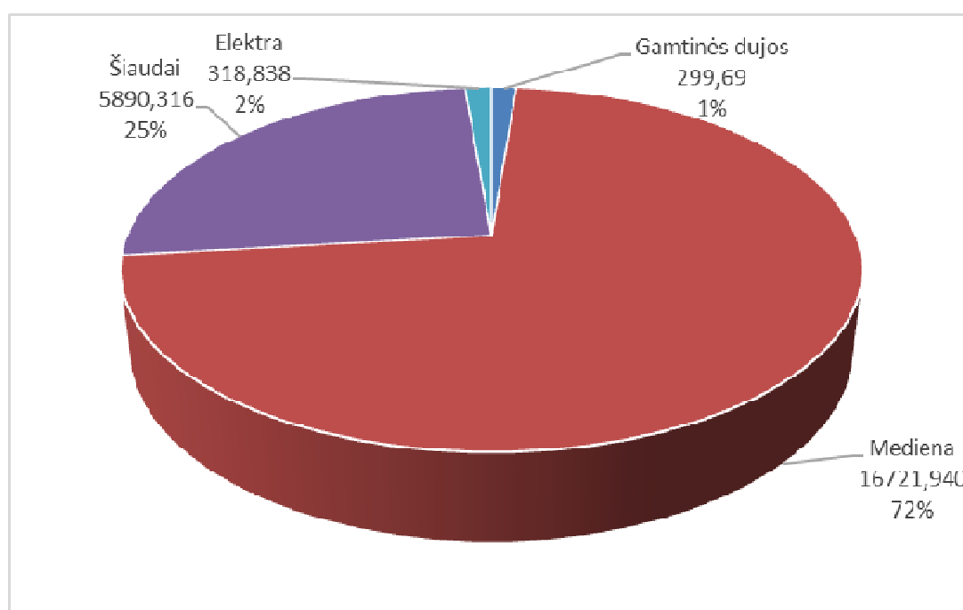
3 pav. 2023 m. UAB „Šakių šilumos tinklai“ sunaudoto kuro balansas, MWh (proc.)
