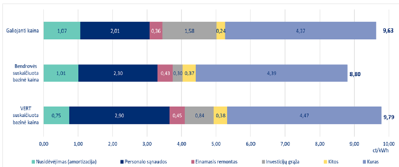
4 pav. UAB „Šakių šilumos tinklai“ šilumos bazinės kainos, ct/kWh be PVM
