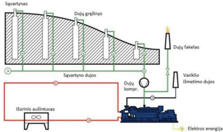
16 pav. Kogeneracinės jėgainės veikimo schema
