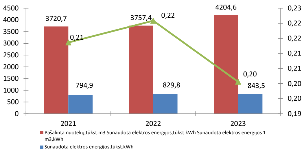
Surinktų nuotekų kiekio ir sunaudotos elektros energijos kitimas
