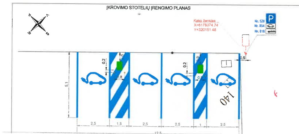
4,5 paveikslas. Elektromobilių įkrovimo stotelių matmenys, ir įrengimo vietos.
