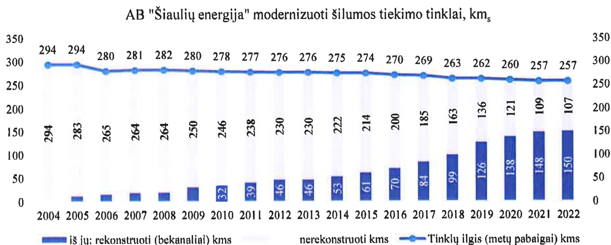
6 pav. AB „Šiaulių energija“ modernizuoti šilumos tinklai
